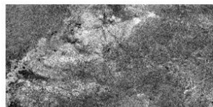
Хлорит- Эпидот
