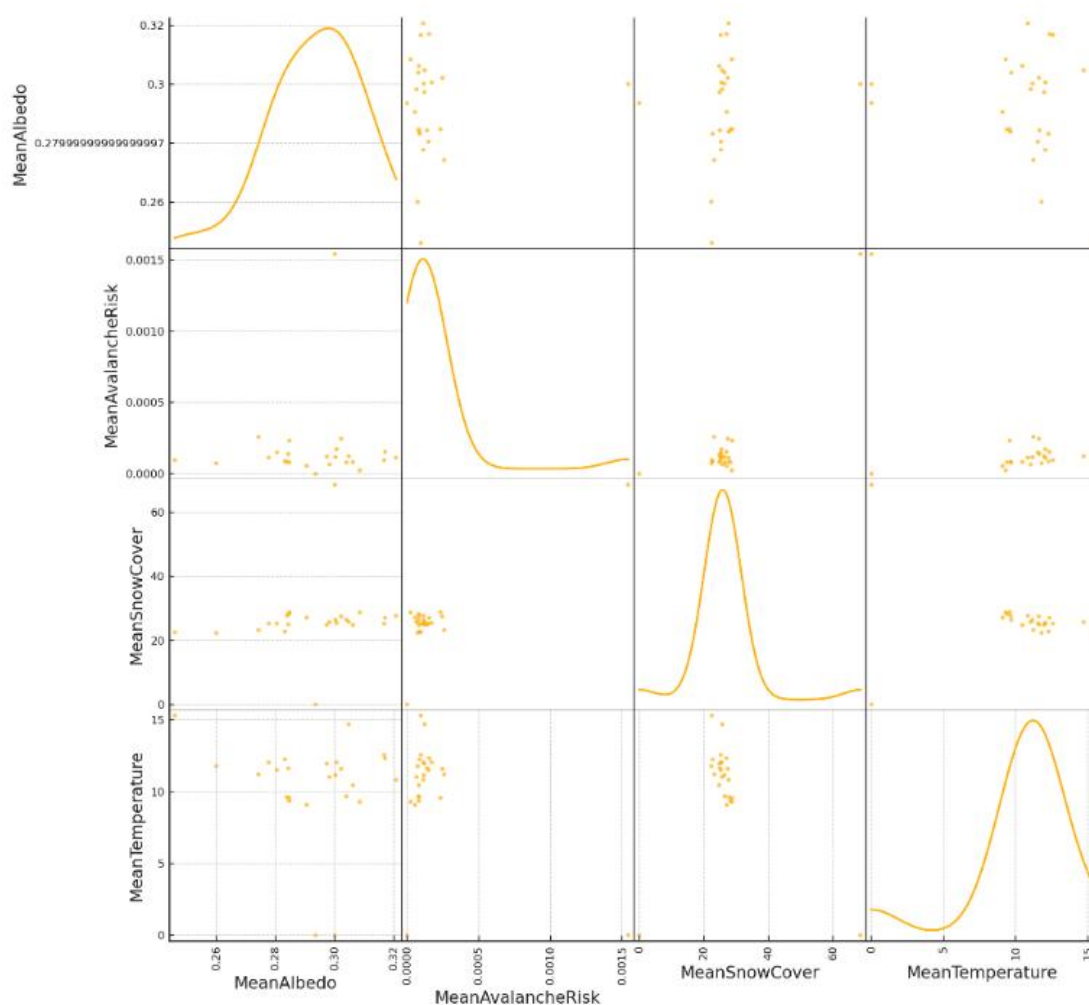
Рисунок-5. График матрицы рассеяния
