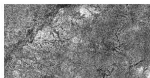
Серицит Мусковит
