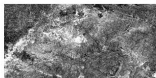
Кальцит
