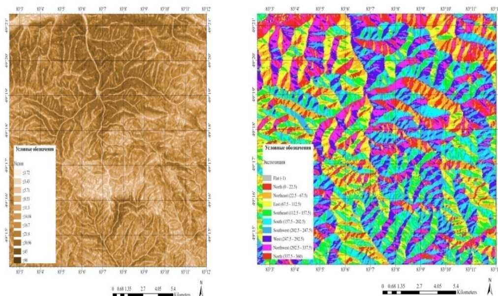
Рисунок 1 - Фрагменты уклона рельефа (слева) и рассчитанной экспозиции склона (справа) для территории ВКО.
