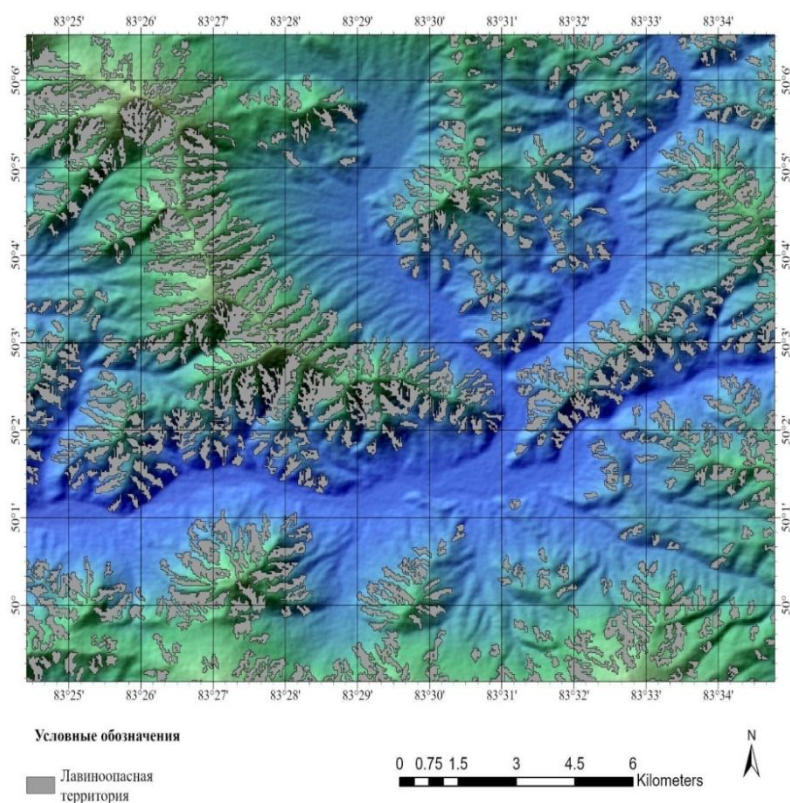
Рисунок 4 - Пример рассчитанных лавиноопасных территорий на ВКО
